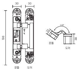
[YHI-016 경첩 좌/우 옵션 선택]
