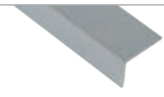
AWM-005 금속 마감 몰딩 [실버] (19×10×2,400)
