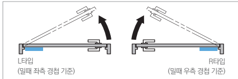
[YHI-021 히든 경첩] * 적용 가능 핸들 - 마그네틱, 데드락, 풀 핸들만 가능
